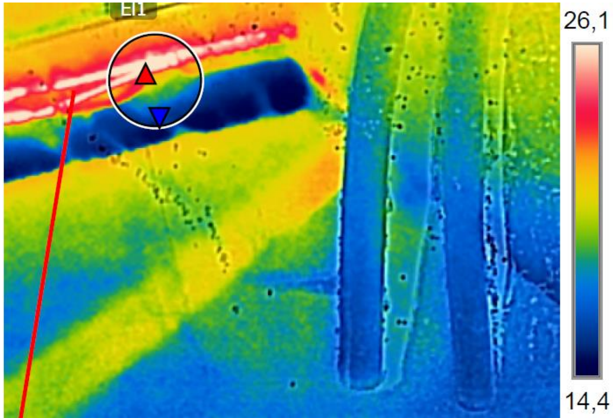
Ongeïsoleerde c.v. leiding.
